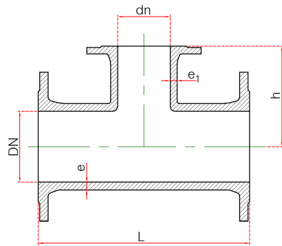
สามทางหน้าจาน 3 ด้าน
