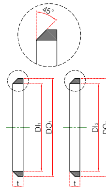
แหวนยาง
