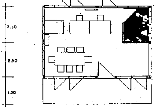
FLOOR PLAN (แก้ไข ๓) (แปลนพื้น)
