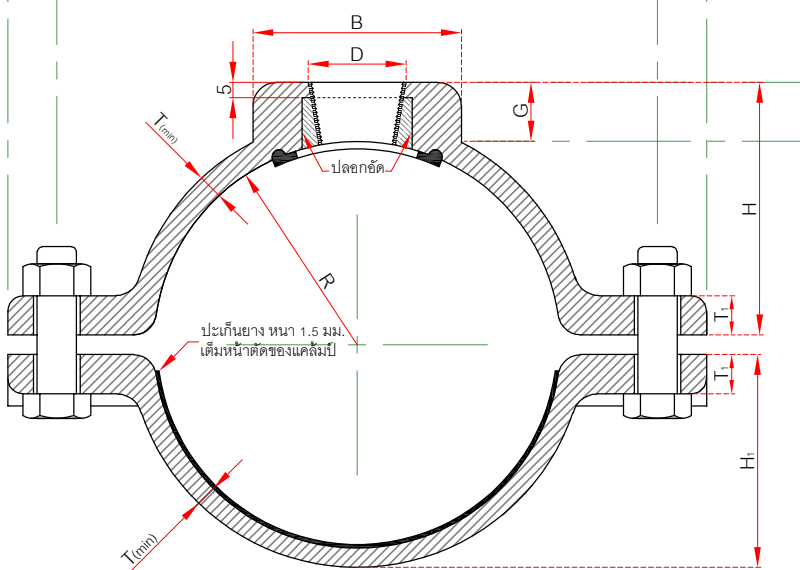
แคล้มปรีดท่อ
