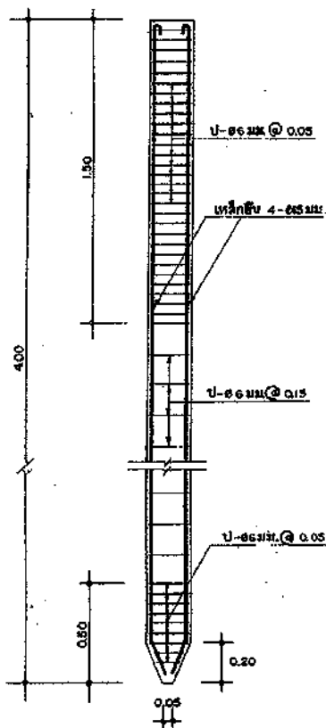
เหล็กรวมคานกริด เสร็จเสริมเหล็ก. ขนาด 0.26 x 0.26 x 4.00
