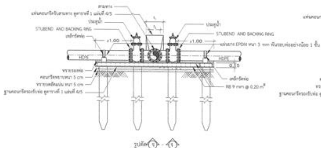
ฐานและแผ่นคอนกรีตเสริมเหล็กสำหรับจุดต่อท่อ HDPE สำหรับประตูปืน 2 ตัว และเสาเข็มที่แยกออกเป็นท่อนยึดขึ้น
