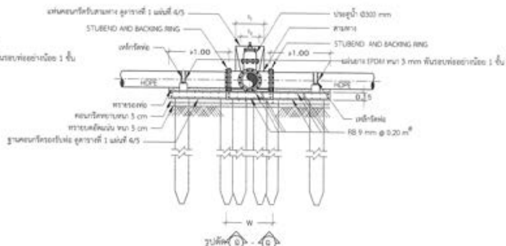
ฐานและแผ่นคอนกรีตเสริมเหล็กสำหรับจุดต่อท่อ HDPE สำหรับเสาเข็มที่แยกออกเป็นท่อ HDPE
