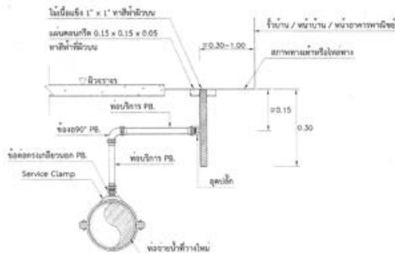
แบบที่ 1 การฉีกวางท่อแยกในฝั่งเดียวกันกับท่อจ่ายน้ำที่วางใหม่
