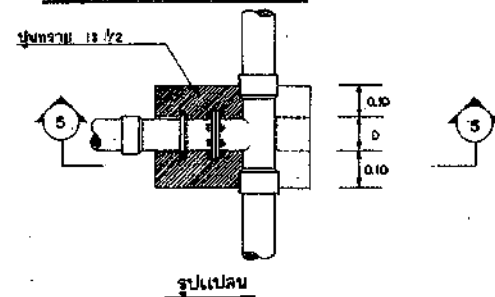
รูปแปลน
