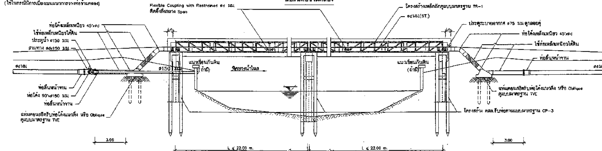
รูปด้านข้าง
