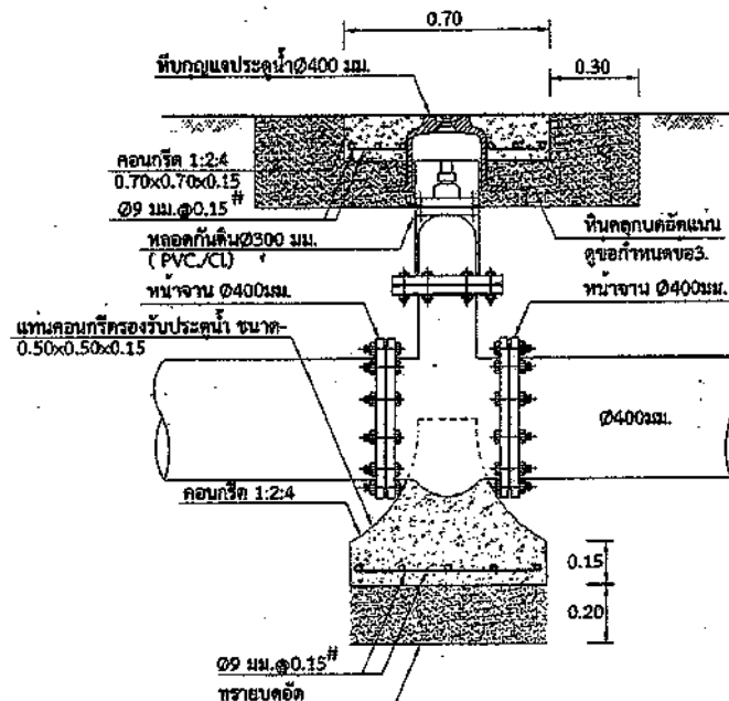
รูปแบบการติดตั้งประตุน้ำ ท้าวจานและหลอดกันดิน
