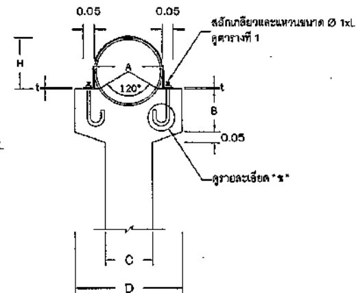
รายละเอียด "ก"
