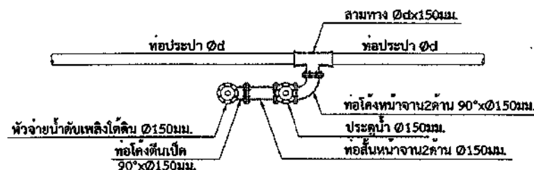
รูปคคก-ก
