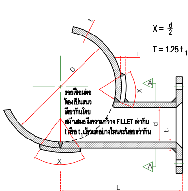
สามทางระบายน้ำ
