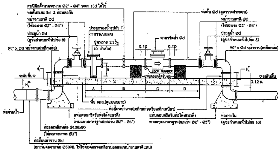
แบบมาตรฐานการติดตั้งมาตรวัดน้ำ ขนาด 2" - 16"
