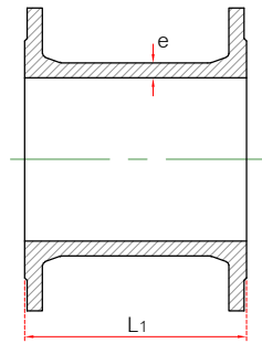
ท่อน้ำจาน 2 ด้าน
