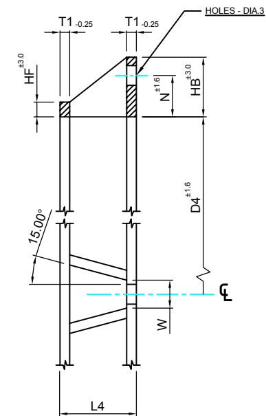
แหวนยึดรั้ง
