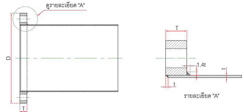
หน้าจานสำหรับงานเชื่อม การเชื่อมหน้าจาน
