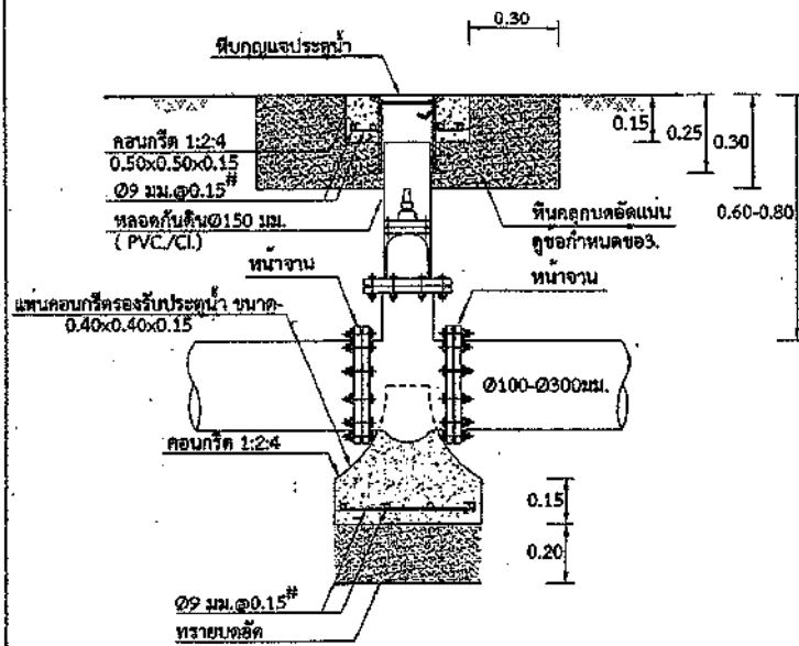
รูปแบบการติดตั้งประตุน้ำ ท้าวจานและหลอดกันดิน
