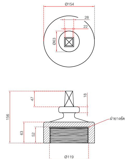
ฝาครอบหัวดับเพลิง (เหล็กหล่อ / เหล็กหล่อเหนียว)
