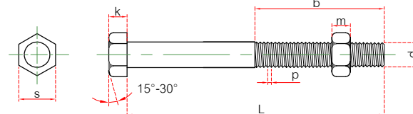
สลักเกลียวและแป้นเกลียว
