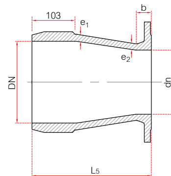
ทอลดน้ำจานด้านลด
