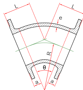
ท่อนํ้าลายเรียบ 2 ด้าน
