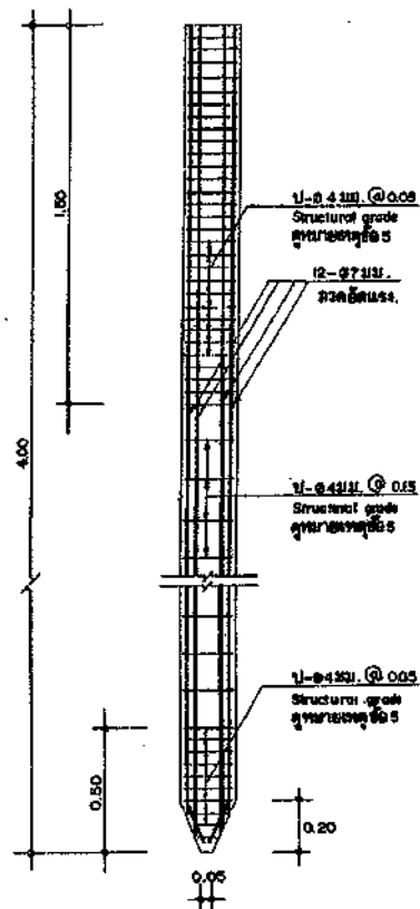
เหล็กรวมคานกริด ยึดแรง ขนาด 0.26 x 0.26 x 4.00
