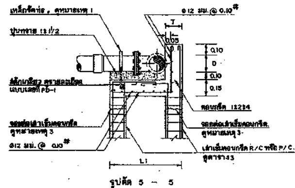
รูปตัด 5 - 5
