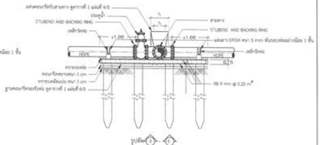
ฐานแผ่นท่อนคอนกรีตรองรับจุดต่อท่อ HDPE สำหรับประตุน้ำ 1 ตัว และฐานทางที่ขยายออกเป็นท่อนิดสั้น
