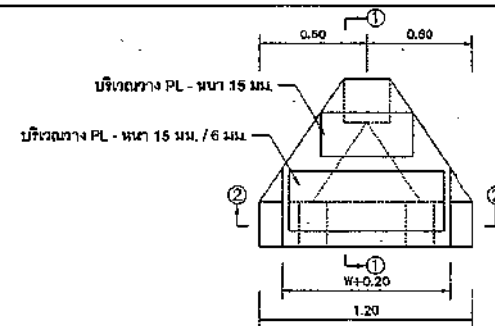
แปลนโครงสร้าง ค.ส.ล.
