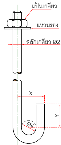
สลักเกลียวรูปตัว J
