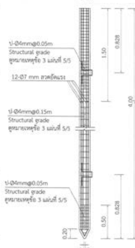
รายละเอียดเสาเข็ม P/C ขนาด 0.26x0.26x4.00 m
