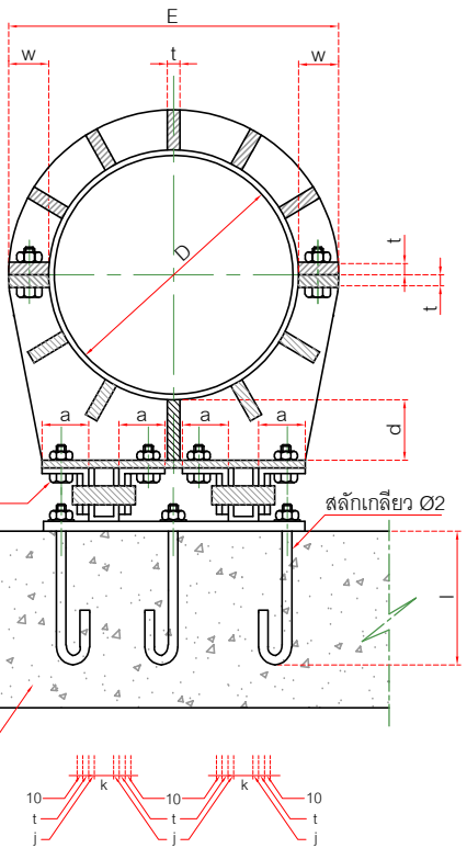
รูปตัด B-B
