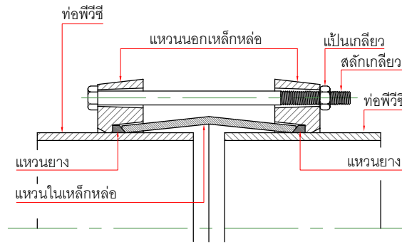
ข้อต่อยึบล็อท
