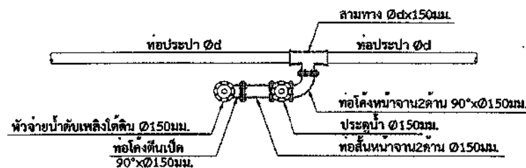
รูปคคก-ก
