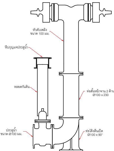
ชุดประกอบหัวดับเพลิง
