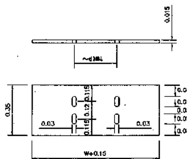
รายละเอียด (ฉ) (Free Support)
