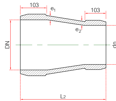
ท่อลดปลายเรียว
