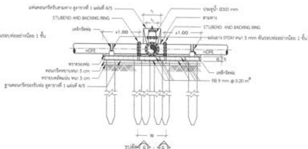
ฐานและแผ่นคอนกรีตรองรับจุดต่อท่อ HDPE สำหรับเสาเข็มที่แยกออกเป็นท่อ HDPE
