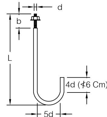
รายละเอียด "ข"
