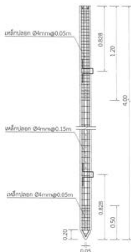
รายละเอียดเสาเข็ม P/C ขนาด 0.15x0.15x4.00 m
