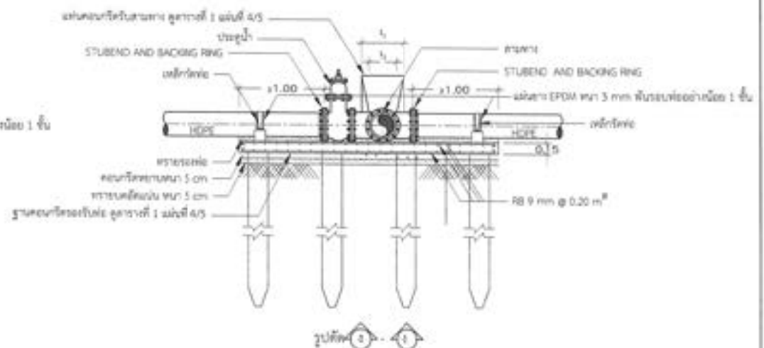
ฐานแผ่นท่อนคอนกรีตรองรับจุดต่อท่อ HDPE สำหรับประตุน้ำ 1 ตัว และฐานทางที่เบี่ยงออกเป็นหน่วยอื่น
