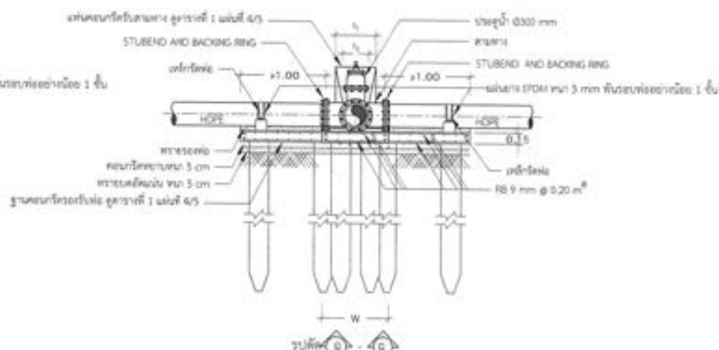
ฐานและแผ่นคอนกรีตเสริมเหล็กสำหรับจุดต่อ HDPE สำหรับเสาเข็มที่แยกออกเป็นท่อ HDPE
