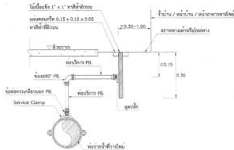
แบบที่ 1 การวางท่อแยกในฝั่งเดียวกันกับท่อจ่ายน้ำที่วางใหม่
