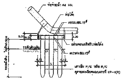
รูปตัด A4 - A4
