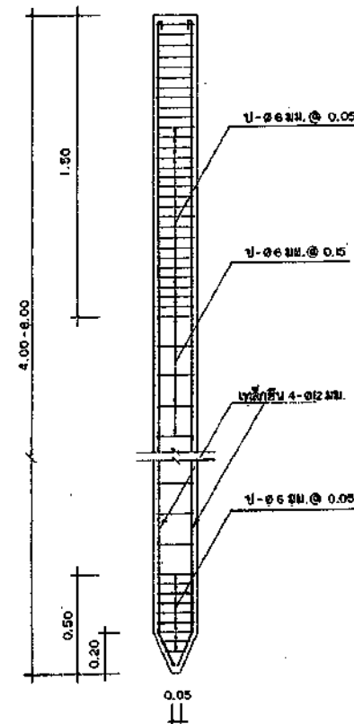
เสาเข็มคอนกรีตเสริมเหล็ก ขนาด 0.18 x 0.18 x 4.00-8.00
