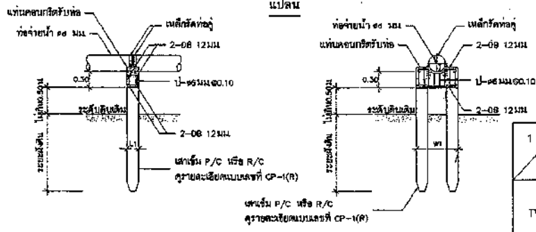
รูปตัด A5 - A5
