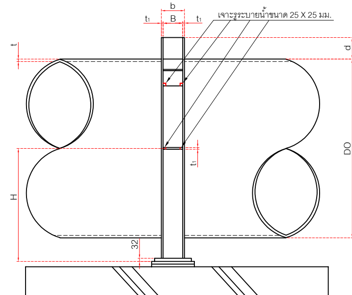
รายละเอียด INSULATING TYPE SHOE แสดงในแบบเลขที่ บ-33 และ บ-34 (FIXED AND MOVABLE SHOES)
