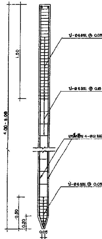
เสาเข็มคอนกรีตเสริมเหล็ก ขนาด 0.16 x 0.16 x 4.00-8.00
