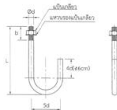
รายละเอียด "ข"
