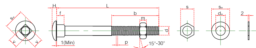
สลักเกลียวและแป้นเกลียว
