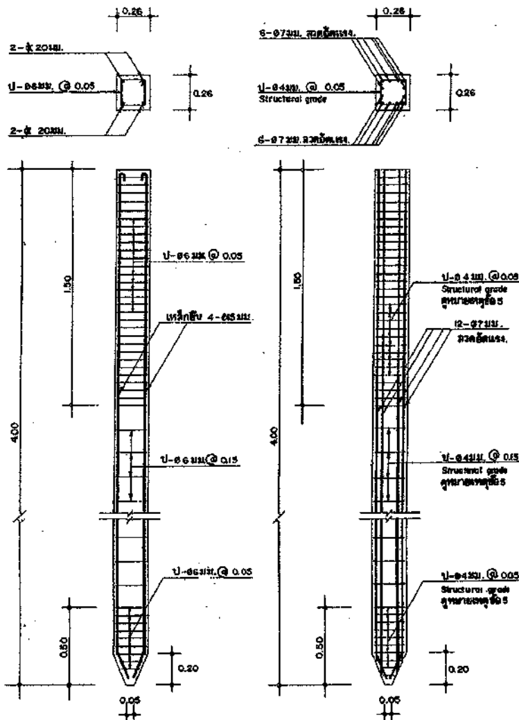
เสาเข็มคอนกรีตเสริมเหล็ก. ขนาด 0.26 x 0.26 x 4.00
