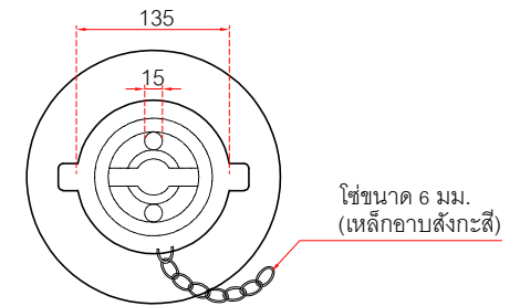
ฝาหีบกุญแจประตูน้ำ
