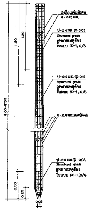
เสาเข็มคอนกรีตอัดแรง ขนาด 0.16 x 0.16 x 4.00-8.00
