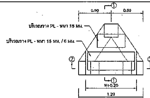
แปลนโครงสร้าง ค.ส.ล.
