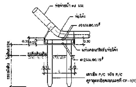
รูปตัด A3 - A3
