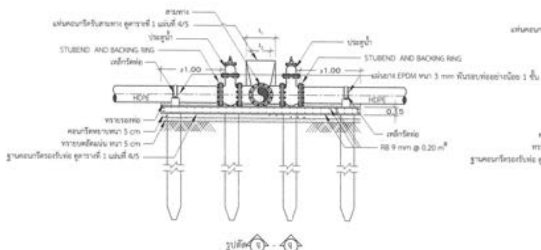
ฐานและแผ่นคอนกรีตเสริมเหล็กสำหรับจุดต่อ HDPE สำหรับประตุน้ำ 2 ตัว และเสาเข็มที่แยกออกเป็นพylonคี่
