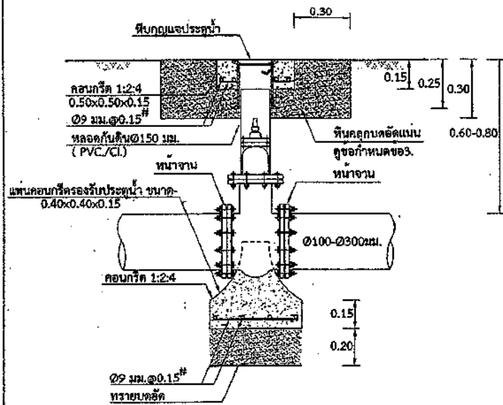
รูปแบบการติดตั้งประตุน้ำ ทึบถูญและหล่อคันทัน
